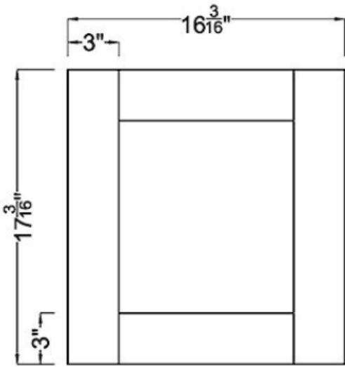
Door x2
