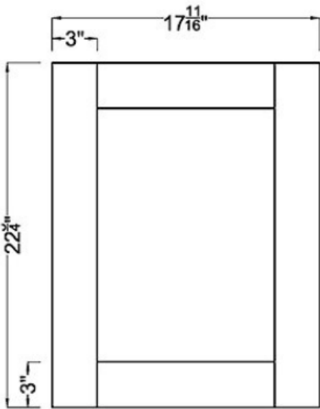
Door ×2
