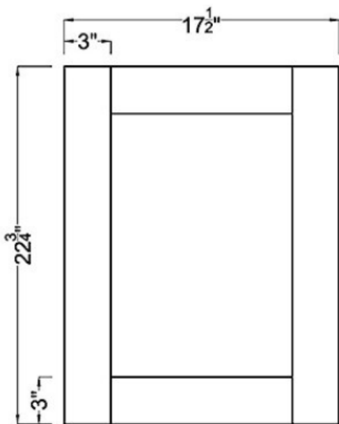
Door ×1
