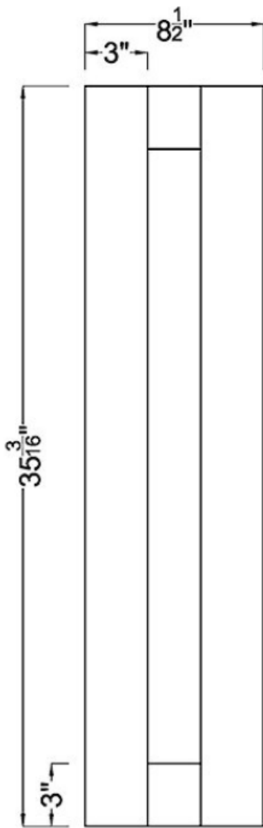
Door x1
