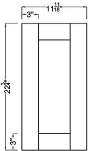
Door ×2
