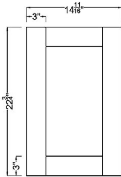
Door ×2
