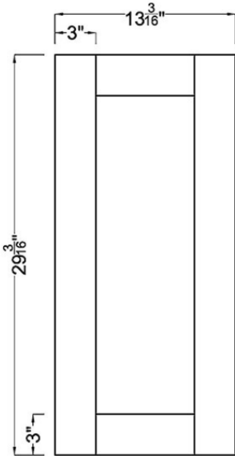
Door x2
