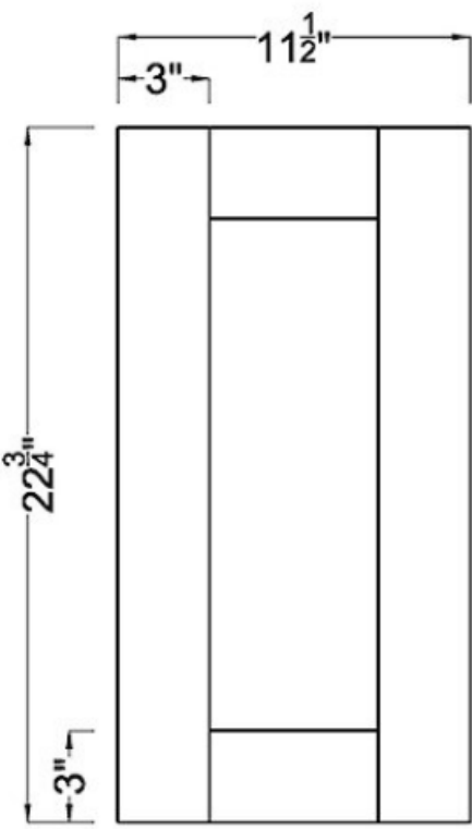
Door ×1
