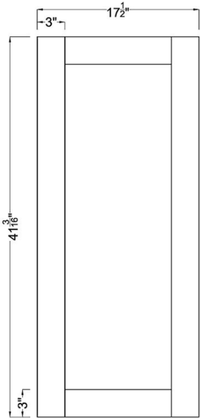
Door x1
