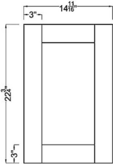
Door x2
