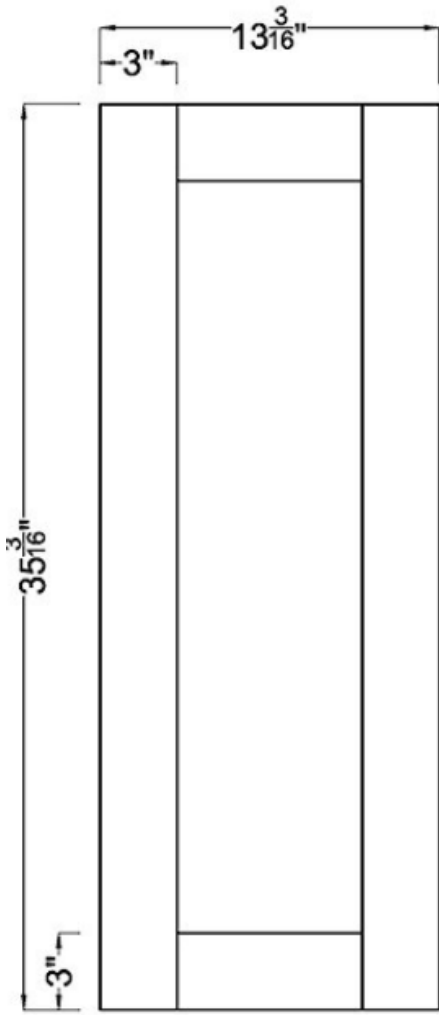
Door x2
