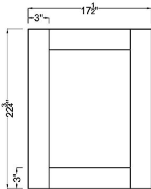
Door ×1
