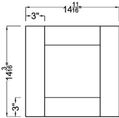
Door x2
