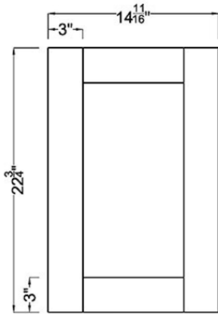
Door x2
