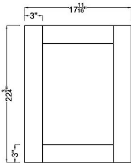
Door x2
