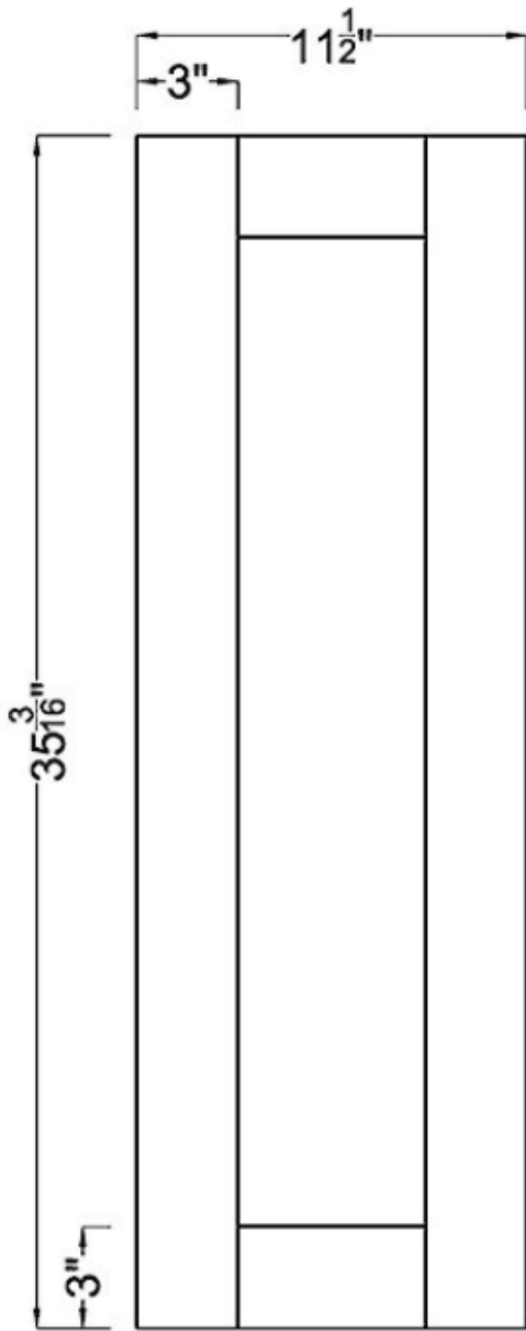
Door x1
