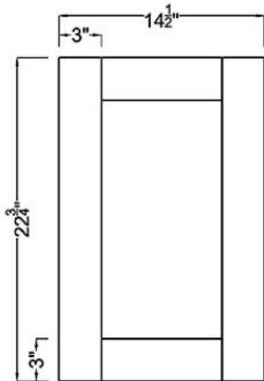
Door ×1
